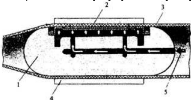
Рис. 12. Приспособление для прижима заплата:
