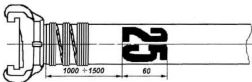
Рис. 4. Дополнительная маркировка рукава на рукавной базе Маркировка наносится на расстоянии 1000÷1500 мм от каждой пожарной соединительной головки краской по трафарету. Для маркировки рукавов допускается использовать краску любого цвета, контрастно отличающуюся от цвета рукава.
